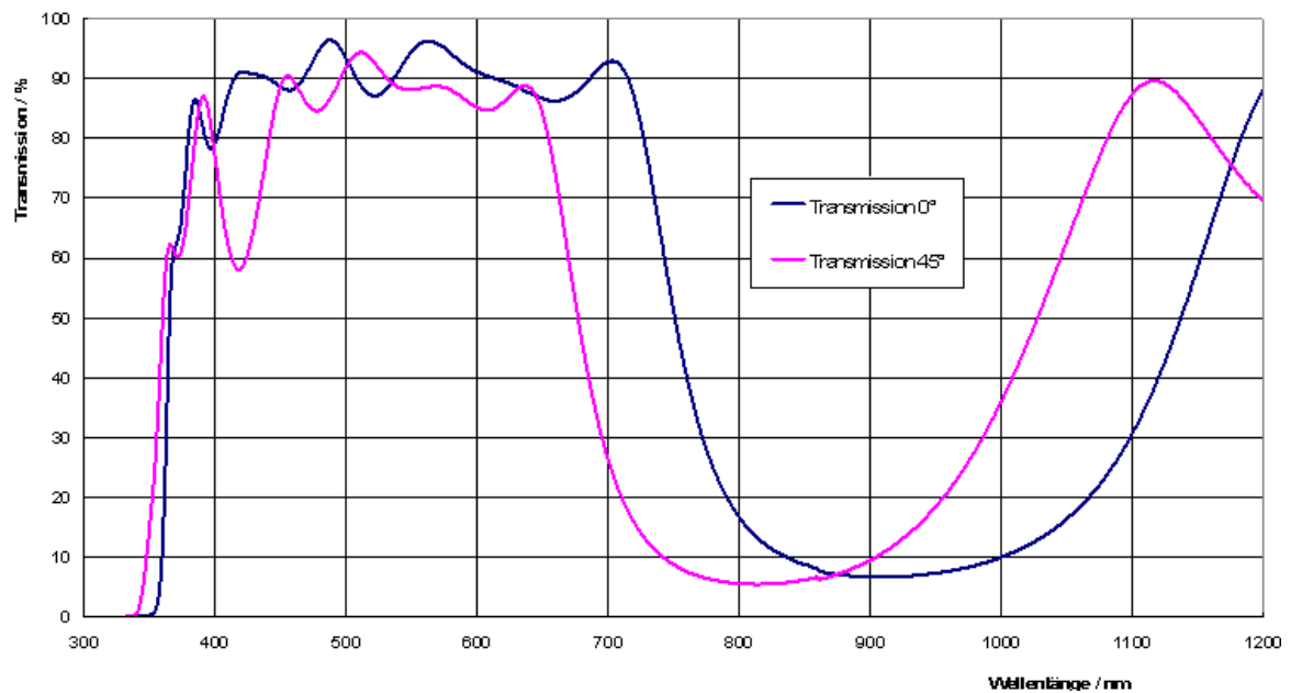
Wärmereflexionsfilter IR3 - Substrat: Borofloat
