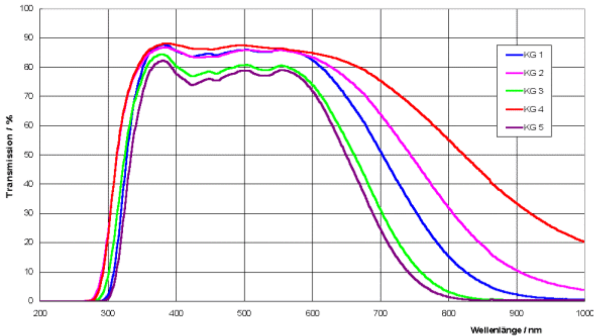
KG - Filter, IR-Bereich, Dicke 3 mm
