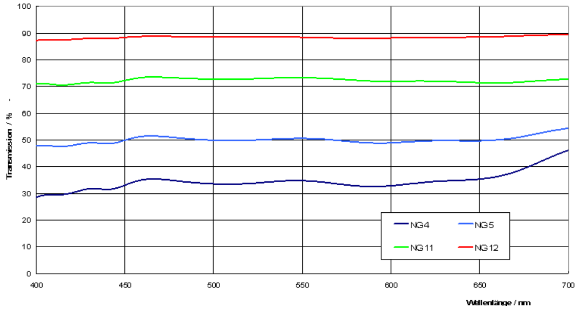
NG - Filter, Dicke 1 mm
