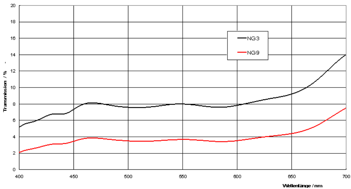
NG - Filter, Dicke 1 mm
