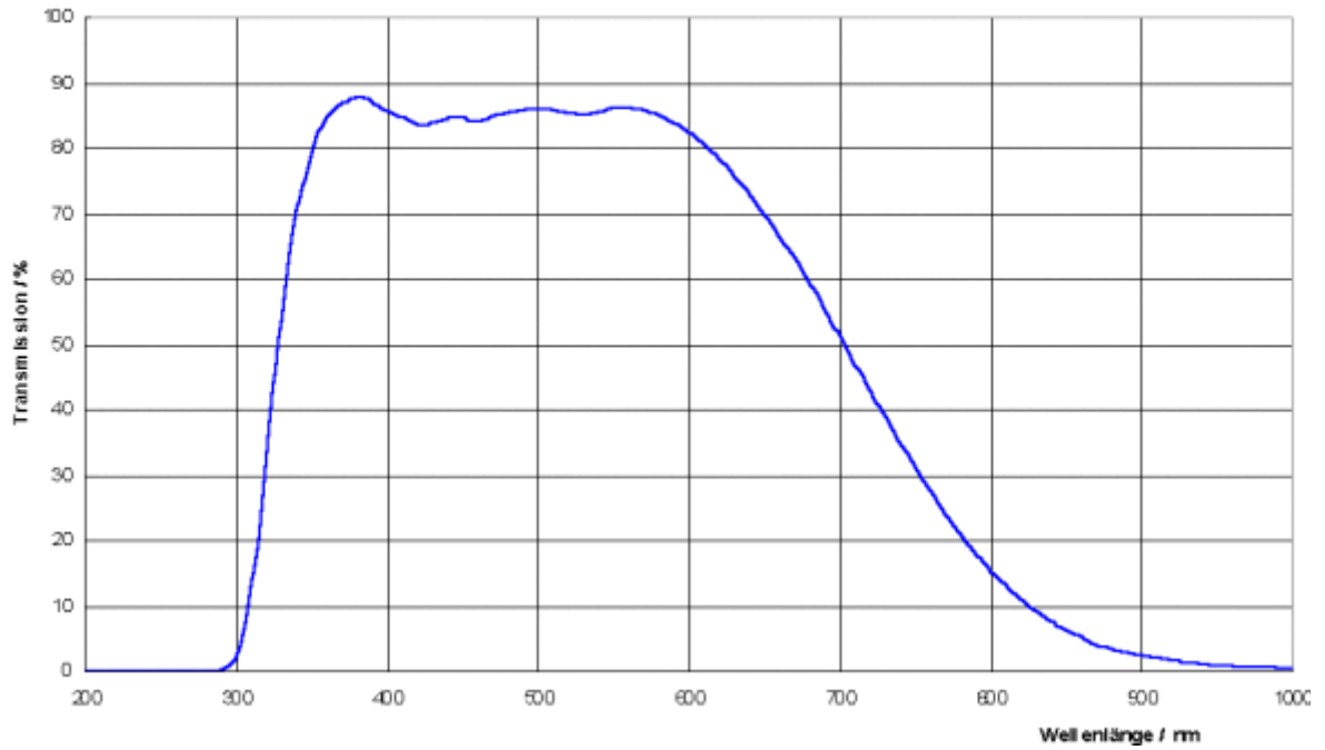
KG 1, IR - Bereich, Dicke 3 mm
