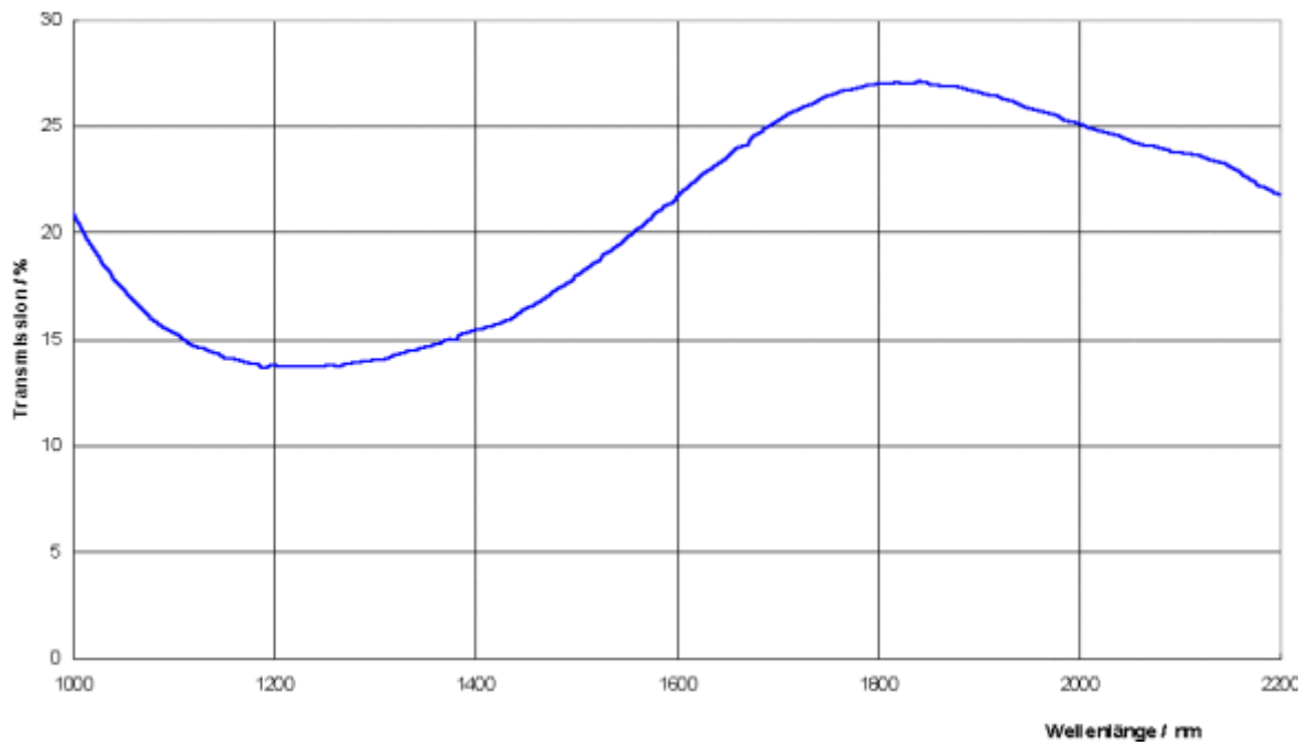
KG4, IR - Bereich, Dicke 3 mm
